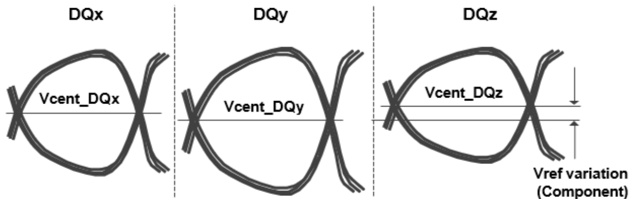
Figure 74. Across Pin Vref DQ Voltage Variation
